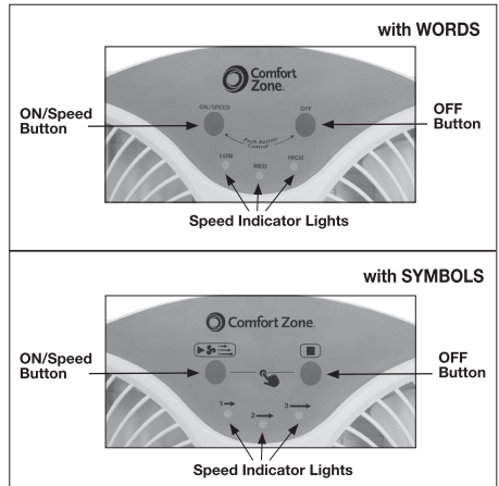
Fig. 8 FAN SPEED CONTROL PANEL
